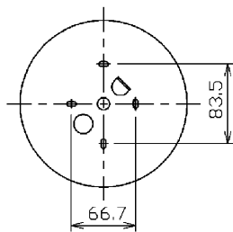
図-2 取り付け寸法図
