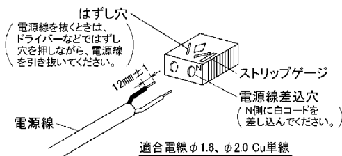
図-3 SL端子台
