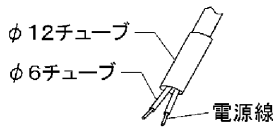
図-1 耐熱保護チューブの取り付けかた
