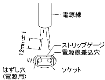
図-2 電源線接続方法
