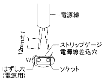
適合電線 \phi 1.6 、 \phi 2.0 Cu単線 図-2 電源線接続方法
