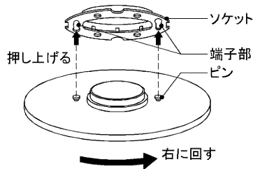
図-4 ランプ取り付け図
