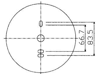
取り付け寸法図
