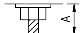
吊りボルト器具内寸法 (A=25mm以下) (図14)
