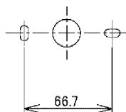
図-2 取り付け寸法図
