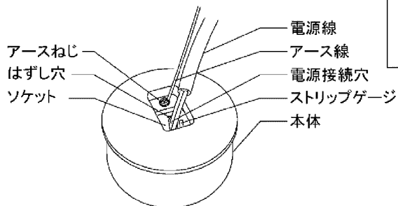
適合電線φ1.6、φ2.0単線 図-4 電源線接続方法
