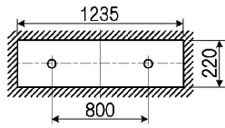
単体取付
