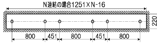
連結取付
