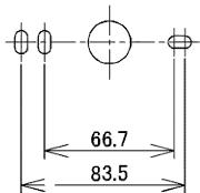
図-3 取り付け寸法図
