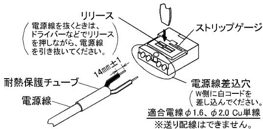
図-5 端子台
