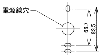
図-2 取り付け寸法図
