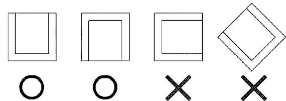
図-4 セード取付方向図
