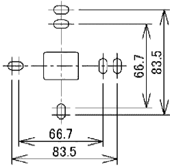
図-2 取り付け寸法図
