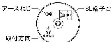
図-4 本体内部
