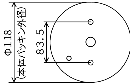
取り付け寸法図
