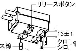
(適合電線φ1.6, φ2.0単線) 第4図
