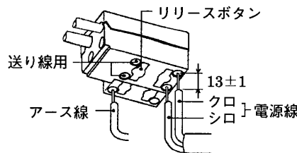
↑押しつける (適合電線 \phi 1.6, \phi 2.0 単線) 電源端子台
