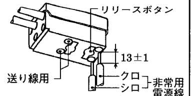
(適合電線 \phi 1.6, \phi 2.0 単線) 非常用電源端子台
