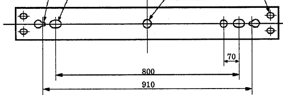
背面仕様図
