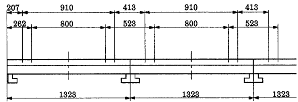
連結寸法図
