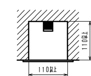
<密閉直付の場合>
