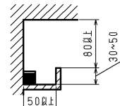
<床置取付の場合>
