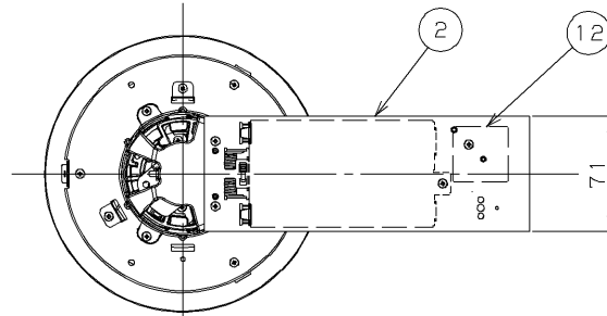
埋込み穴寸法 取付け可能な天井厚: 3mm~25mm
