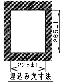
取付け図
