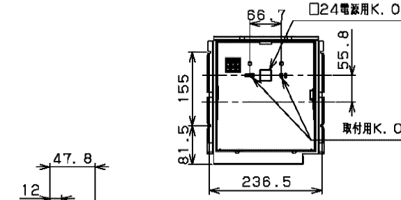
取付け図
