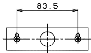
(器具の取付け寸法)
