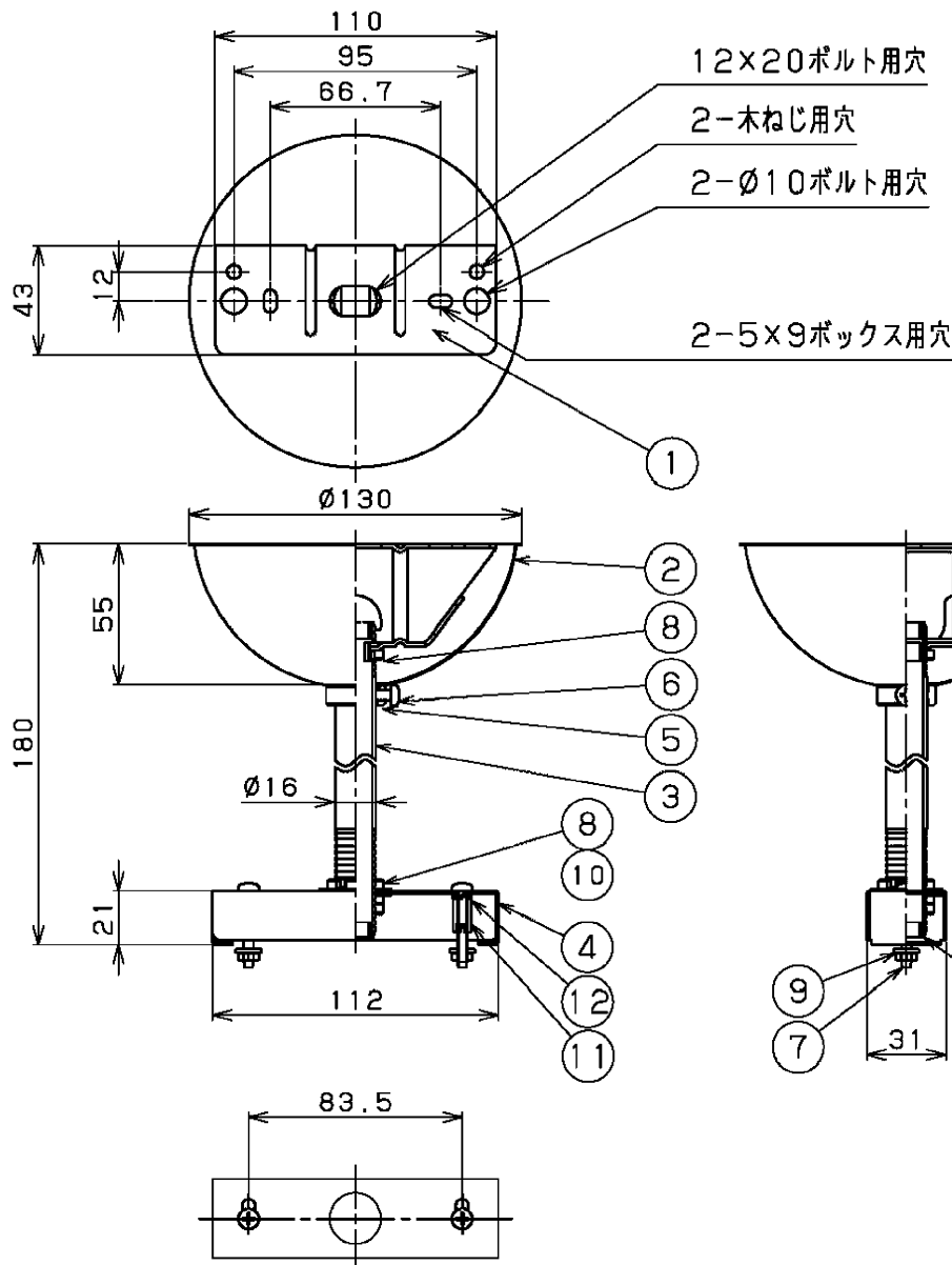
(器具の取付け寸法)
