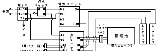
結線図
