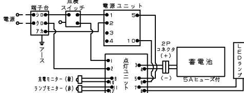
結線図
