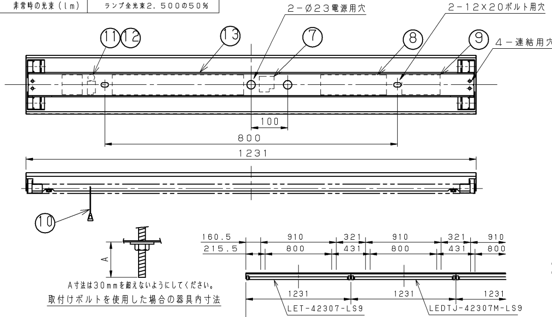
直付け連結使用例
