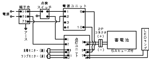
結線図
