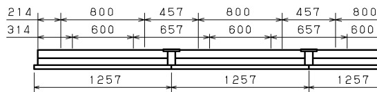
連結使用例
