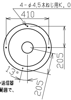
取付けピッチ寸法図
