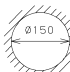
埋込み穴寸法 天井取付け厚さ: 3mm~25mm
