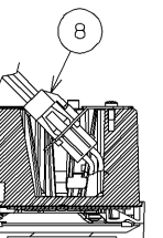
コネクタで電源ユニットとLEDユニットを接続します。
