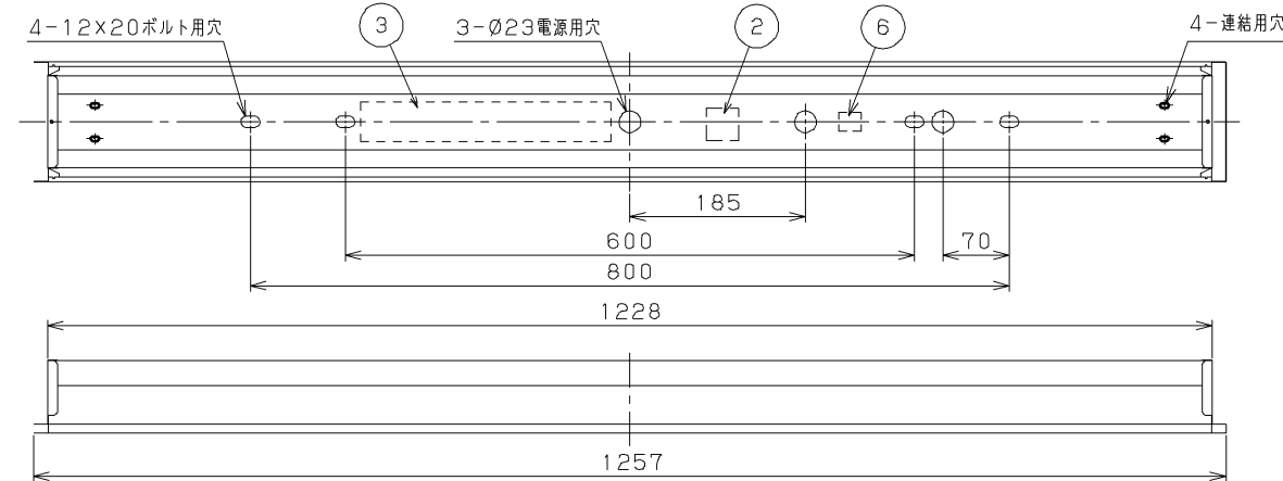
N連結の場合 1257×N-20 埋込み寸法
