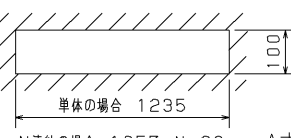
単体の場合 1235 N連結の場合 1257×N-20 埋込み寸法
