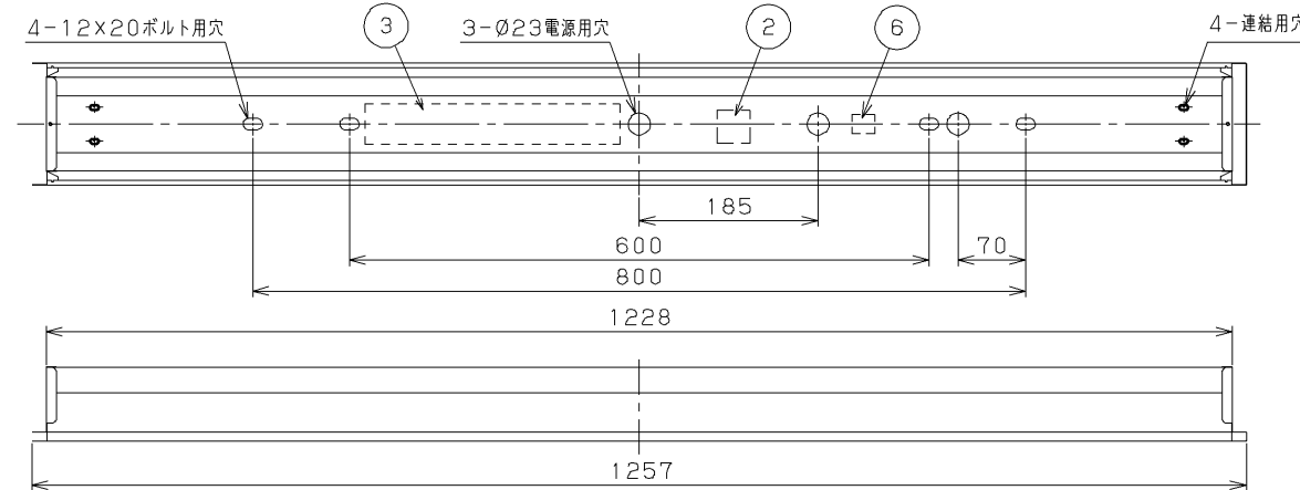
単体の場合 1235 N連結の場合 1257×N-20 埋込み寸法
