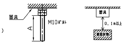
器具取り付けボルトを使用した場合の器具内寸法 ※A寸法は、60mm以下にしてください。
