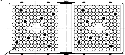
器具取り付けボルトを使用した場合の器具内寸法 ※A寸法は、60mm以下にしてください。
