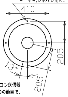
取付けピッチ寸法図 4-φ4.5木ねじ用K.0
