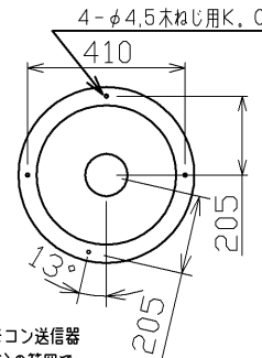
取付けピッチ寸法図
