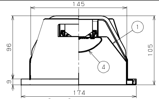
【基本特性】
