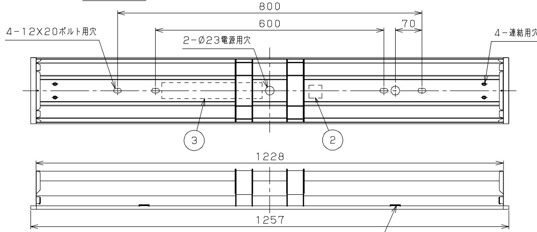
連結使用例
