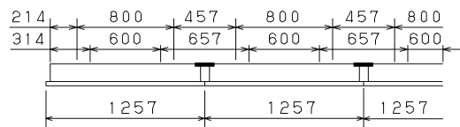
連結使用例
