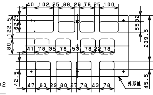
配線穴寸法
