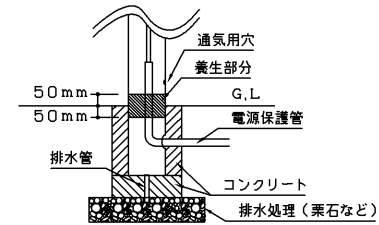
コンクリート施工の場合
