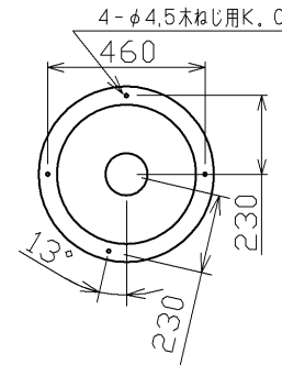
取付けピッチ寸法図
