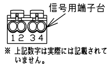
端子台が上向きの配置
