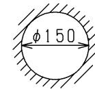
埋込み穴寸法 天井取付け厚さ:5mm~25mm
