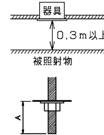
取付けボルトを使用した場合の器具内寸法
