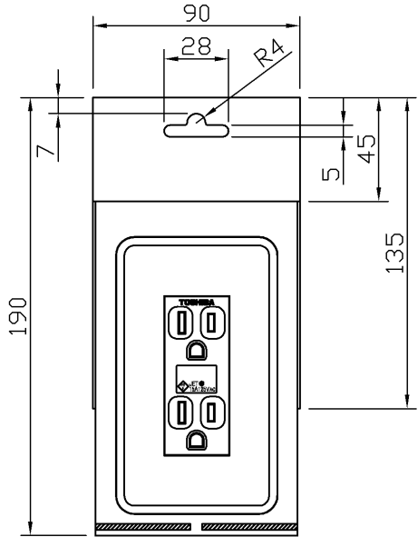
バック寸法
