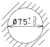
埋込み穴寸法 天井取付け厚さ：5mm~25mm
