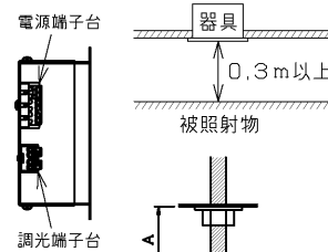
器具取付けボルトの器具内寸法
