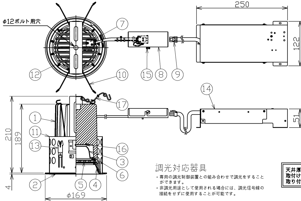
埋込み穴寸法 天井厚さが5mm～25mm
