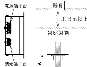
器具取り付けボルトの器具内寸法
