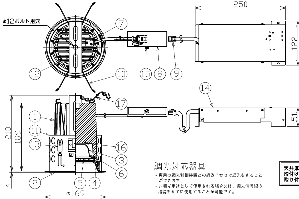
埋込み穴寸法 天井厚さ：5mm～25mm
