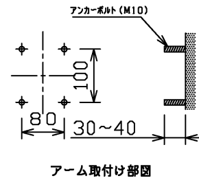
アーム取付け部図
